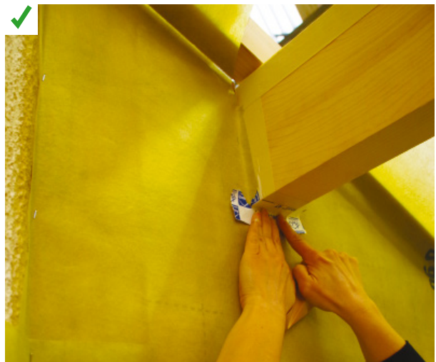
La membrane d'étanchéité à l'air est traversée par un élément de charpente. L'étanchéité à l'air de ce point singulier est traitée grâce à du ruban adhésif approprié qui permet de fixer la membrane sur le pourtour de la poutre. ©AQC
