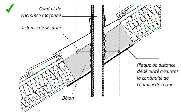
Pour les conduits maçonnés, l'espace créé par le respect de la distance de sécurité ne peut pas être composé d'un matériau isolant. Le respect des règles de l'art entraîne donc un pont thermique pour ce cas précis.. ©AQC
