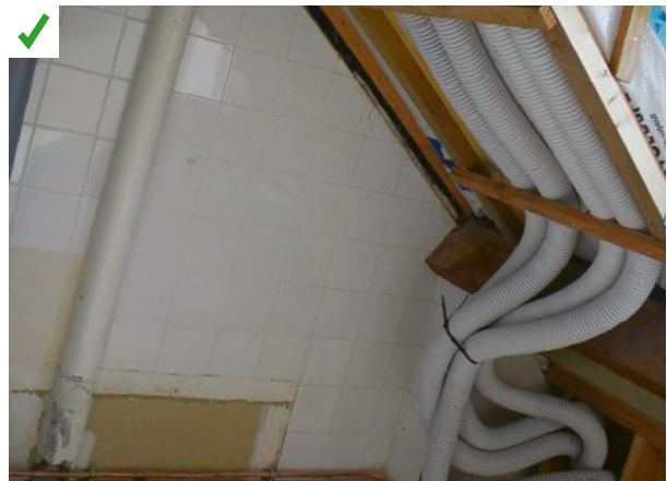
Création d'un vide technique pour le passage des gaines de ventilation double flux permettant d'éviter le percement de la membrane d'étanchéité à l'air. ©V. Jacquet
