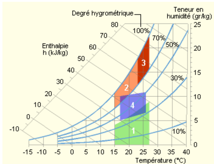
Illustration 16 : Les quatre zones de confort hygrothermique (source : energieplus-lesite.be)
