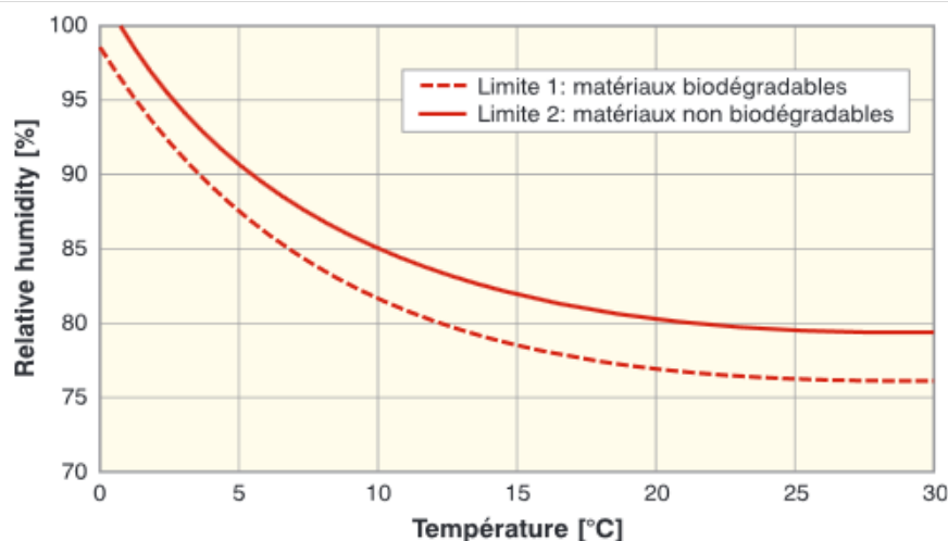
Illustration 14 : Conditions en température et en humidité relative favorables au développement de moisissures (source : [guide ISOLIN, 2010] d'après [logiciel WUFI, 1995])
