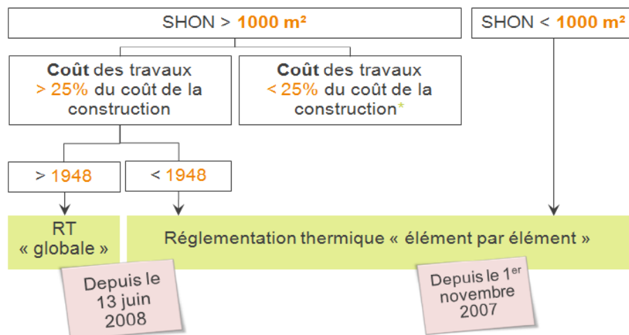
Illustration 3 : Schéma synoptique de la réglementation thermique des bâtiments existants en France (source : Ministère de l'Écologie, site rt-batiment.fr)
