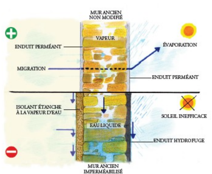
Illustration 7 : Fonctionnement hygrothermique d'un mur ancien rénové ou non (source : [fiches ATHEBA, 2011])
