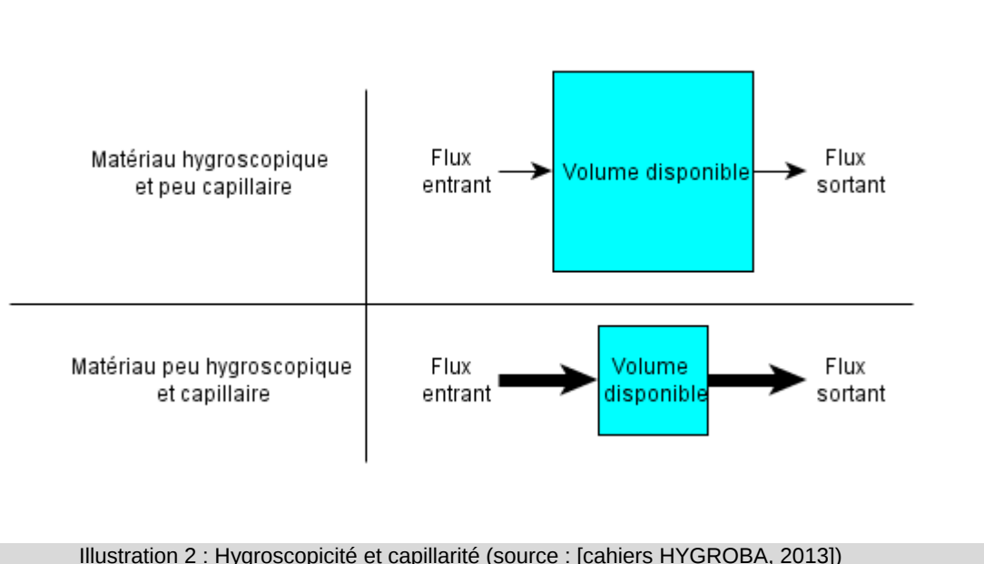
Illustration 2 : Hygroscopicité et capillarité (source : [cahiers HYGROBA, 2013])
