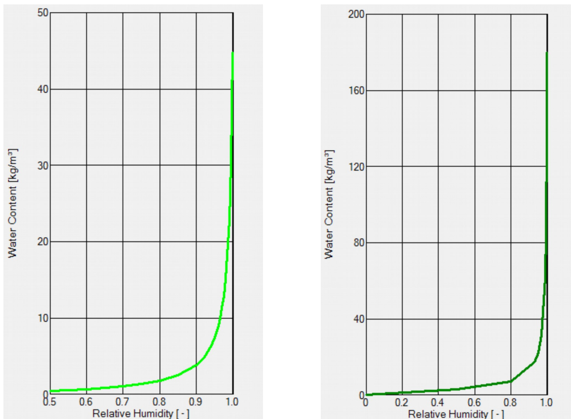
Illustration 1 : Courbes de sorption pour un matériau peu hygroscopique (à gauche, polystyrène extrudé) et pour un matériau hygroscopique (à droite, laine de bois) (source : [logiciel WUFI, 1995])
