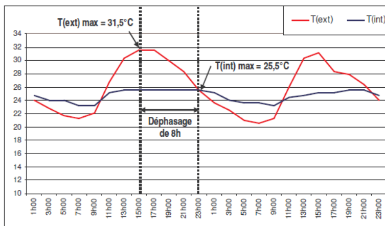
Illustration 5 : Evolution des températures extérieures et intérieures lors de deux journées types d'été pour un bâtiment en pierre de 80 cm d'épaisseur (source : [Pré-BATAN, 2007])
