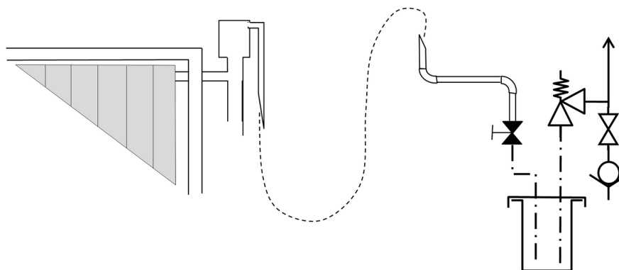
▲ Figure 31 : Purgeur manuel ramené en local technique et branché dans le bidon de récupération
