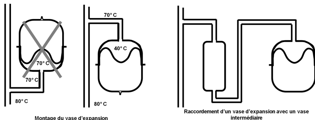
▲ Figure 32 : Raccordement du vase d'expansion
