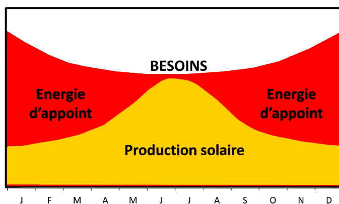
▲ Figure 23 : Evolution de la production solaire au long de l'année
