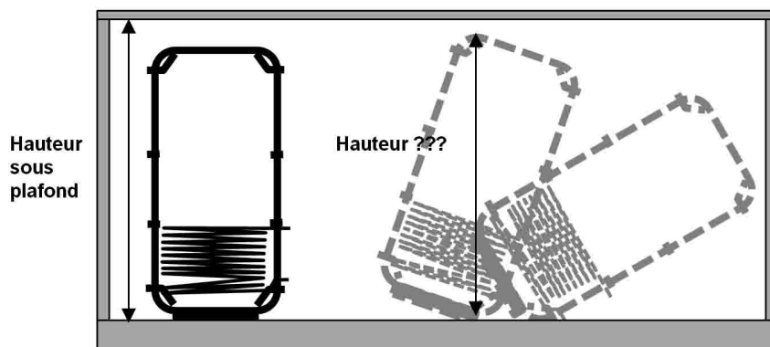
▲ Figure 40 : Contrôle de la diagonale du réservoir
