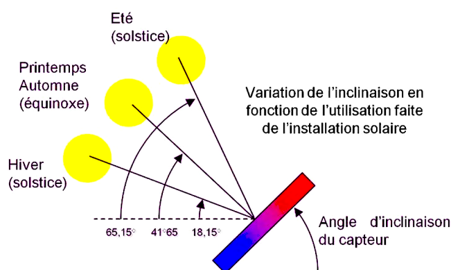
▲ Figure 16 : Hauteur du soleil par rapport à l'horizontale au cours de la journée et de l'année (exemple pour Strasbourg avec une latitude de 48°35')
