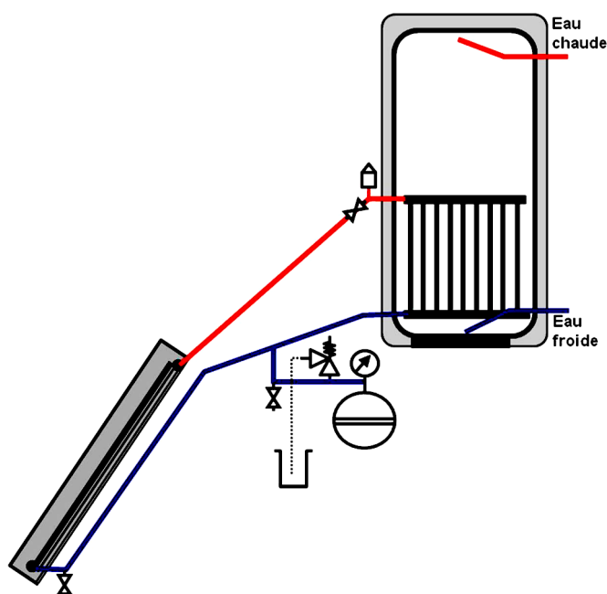
▲ Figure 3 : Schéma de principe d'un thermosiphon à éléments séparés
