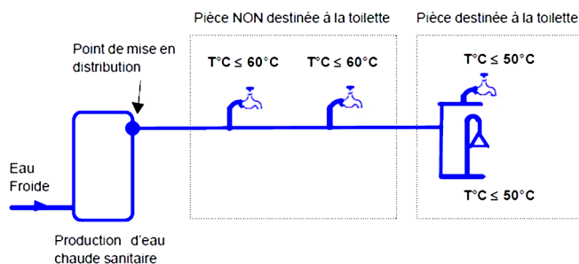
▲ Figure 12 : Prescriptions visant à prévenir le risque de brûlure aux points d'usage
