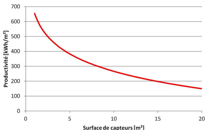
▲ Figure 24 : Influence de la surface de capteurs sur la productivité solaire
