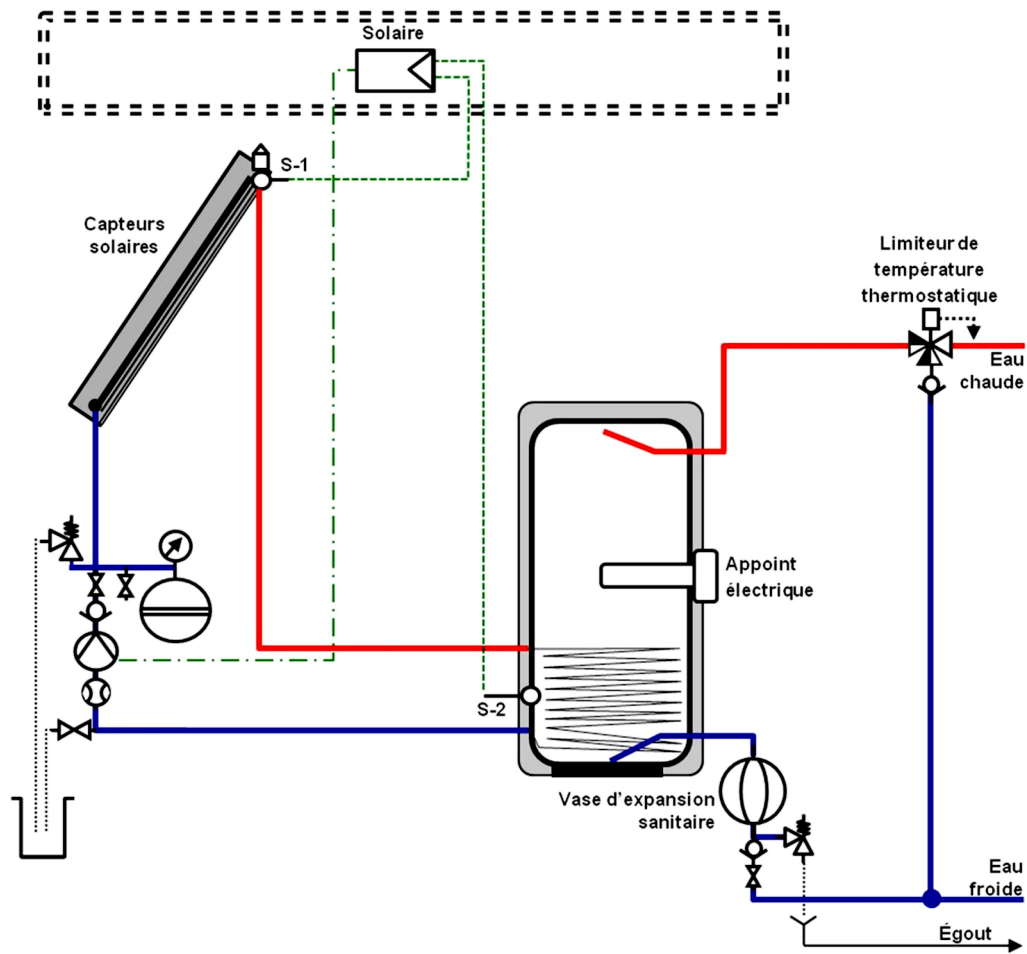
▲ Figure 9 : Schéma de principe de la solution avec appoint électrique intégré
