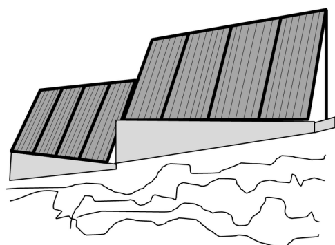
Capteurs plan en deux batteries sur dalle de béton
