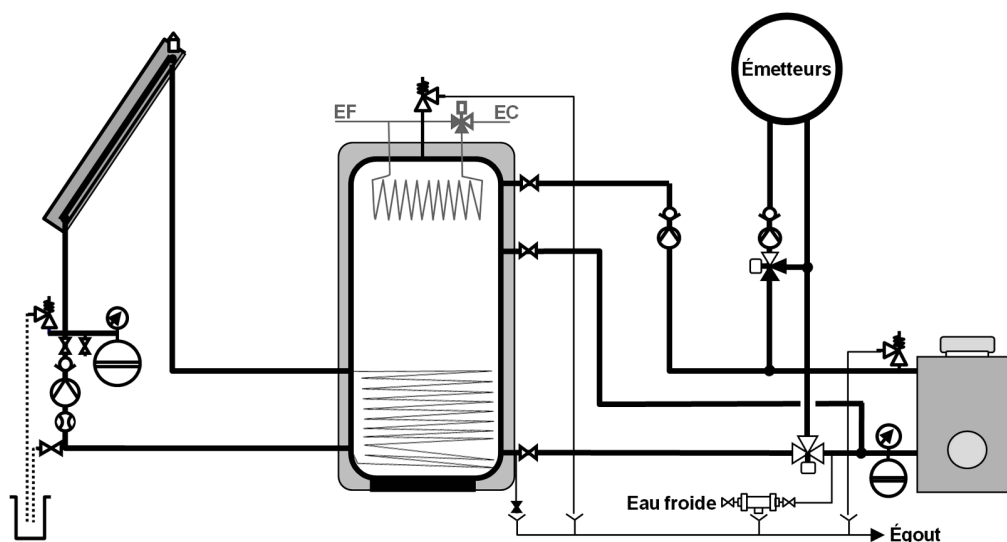
▲ Figure 4 : Schéma de principe d'un raccordement en parallèle
