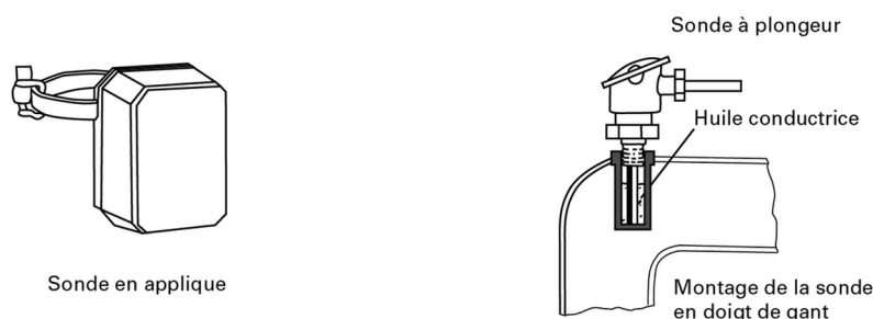
▲ Figure 53 : Les différents types de sonde de mesure de température d'eau
