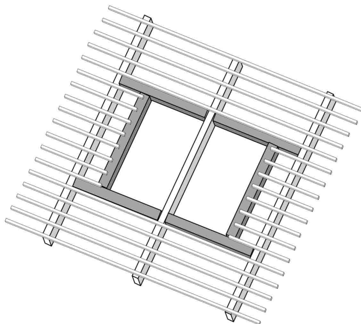
▲ Figure 12 : Réalisation d'un chevêtre pour la pose des capteurs
