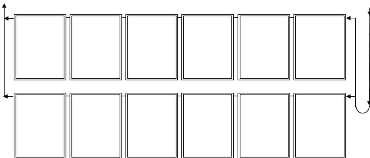
▲ Figure 35 : Raccordement en série et parallèle avec boucle de « Tichelmann »
