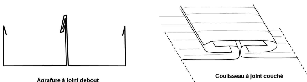
▲ Figure 21 : Exemples de raccordements d'étanchéité
