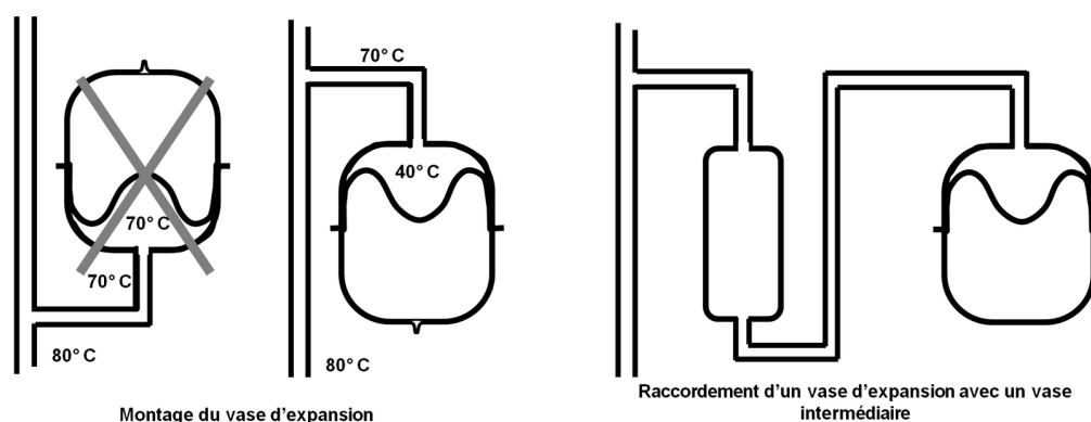
▲ Figure 44 : Raccordement du vase d'expansion
