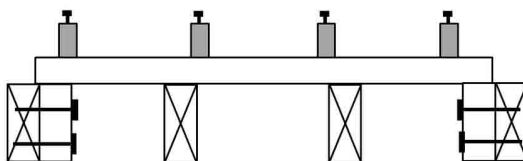
▲ Figure 23 : doublement des chevrons pour renforcement du support des crochets de fixation (face)
