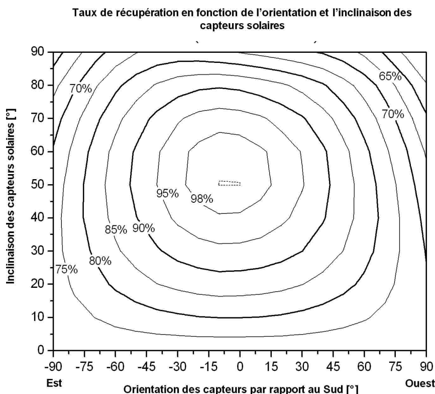
▲ Figure 9 : Taux de récupération d'énergie solaire en fonction de l'orientation et de l'inclinaison des capteurs solaires
