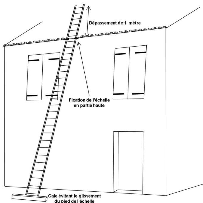
▲ Figure 6 : mise en sécurité d'une échelle
