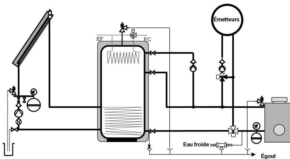
▲ Figure 2 : Schéma de principe d'un raccordement en série (ou réchauffage du retour)
