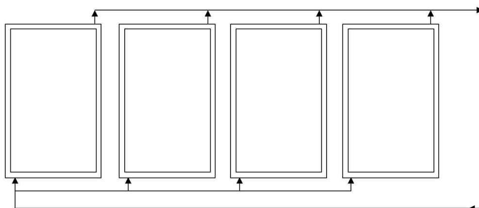
▲ Figure 34 : Raccordement en parallèle de type « Tichelmann »
