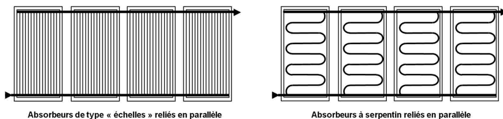
▲ Figure 31 : Exemples de raccordement en parallèle des absorbeurs
