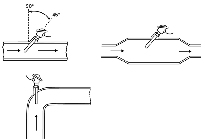
▲ Figure 55 : Exemples de pose de sondes à plongeur
