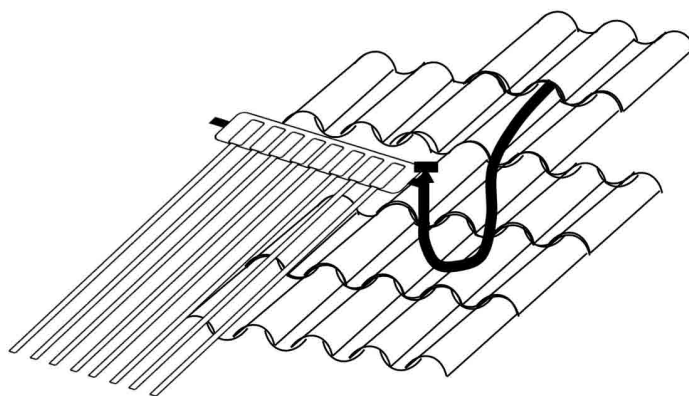
▲ Figure 41 : lyre de dilatation en sortie de capteur à tube sous vide et pénétration de la tuyauterie par une tuile chatière
