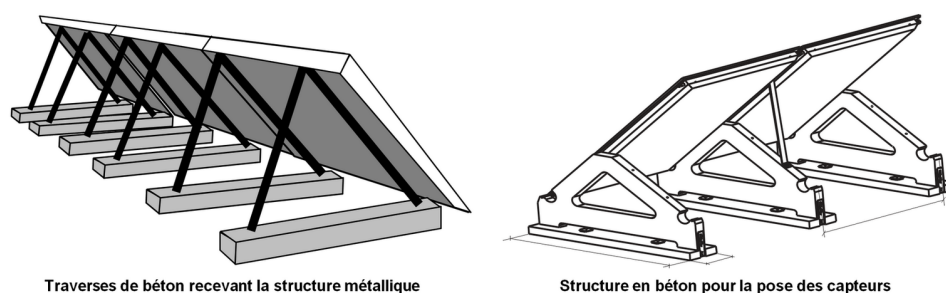
▲ Figure 25 : exemple de lestage de capteurs
