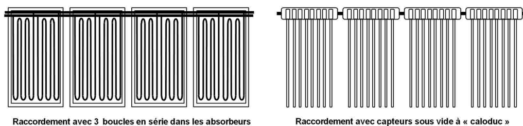
▲ Figure 33 : Différentes particularités de raccordement des absorbeurs
