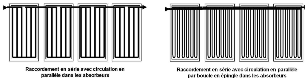
▲ Figure 32: Exemples de raccordement en série des absorbeurs
