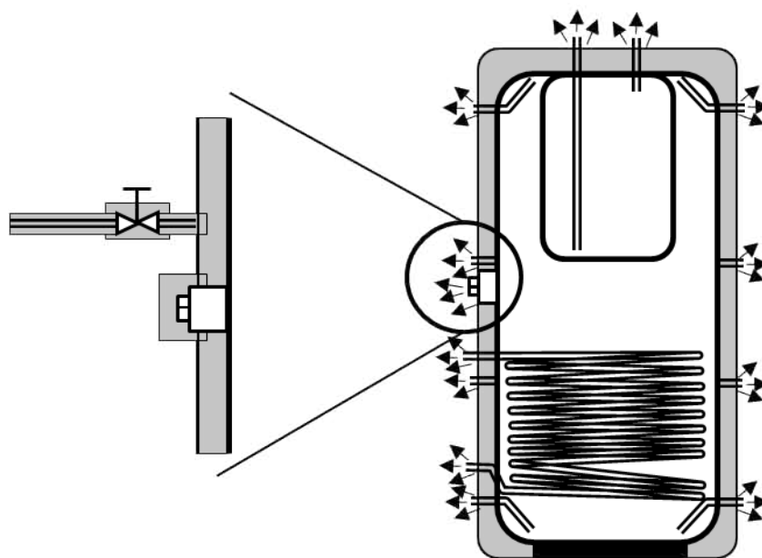
▲ Figure 52 : Tous les piquages raccordés ou non doivent être isolés avec soin
