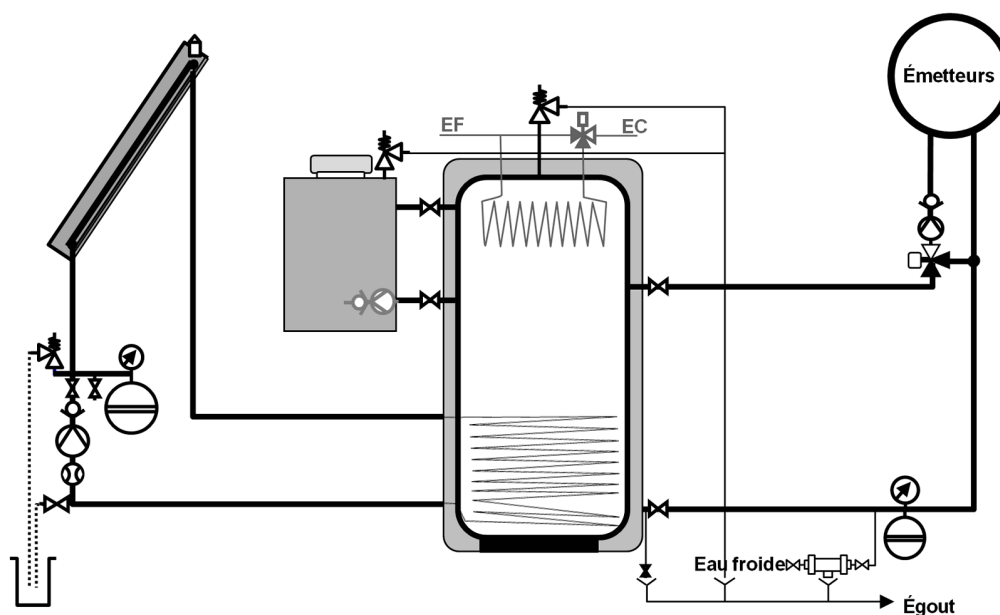
▲ Figure 3 : Schéma de principe d'un raccordement mixte (maintien en température du haut du stockage)
