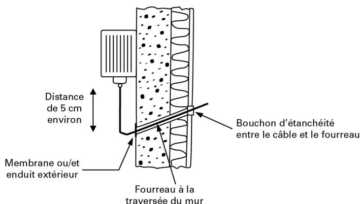
▲ Figure 57 : Exemple de mise en œuvre de la sonde de température extérieure
