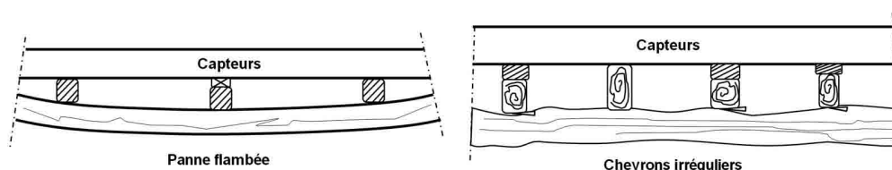
▲ Figure 11 : Calage pour retrouver la planéité de la couverture
