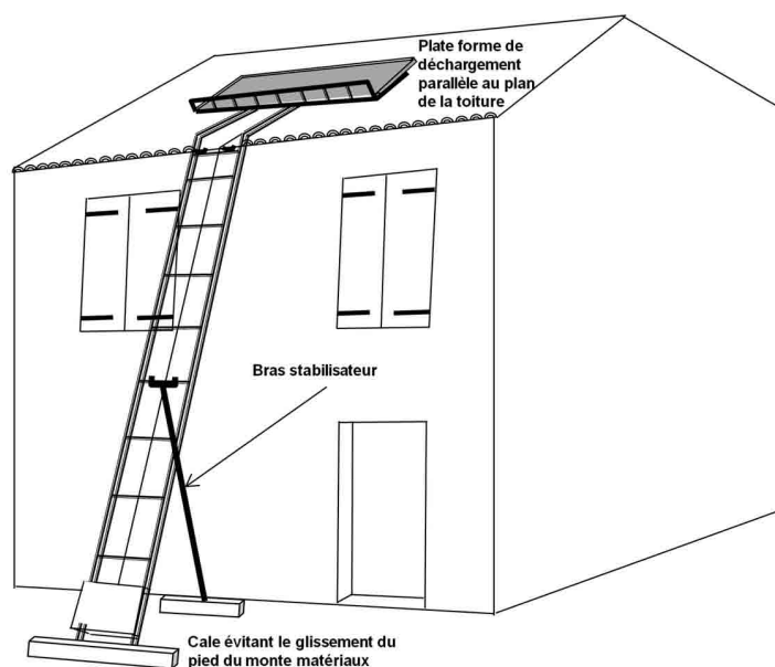
▲ Figure 7 : positionnement du monte-matériaux
