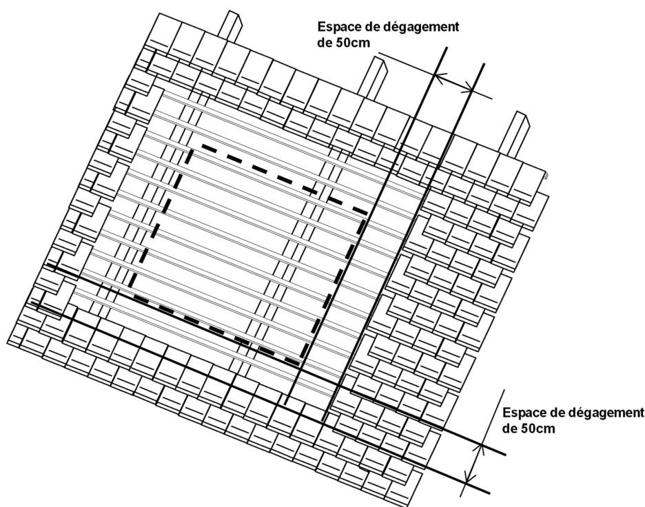
▲ Figure 8 : réservation à prévoir autour de l'emplacement du champ de capteurs
