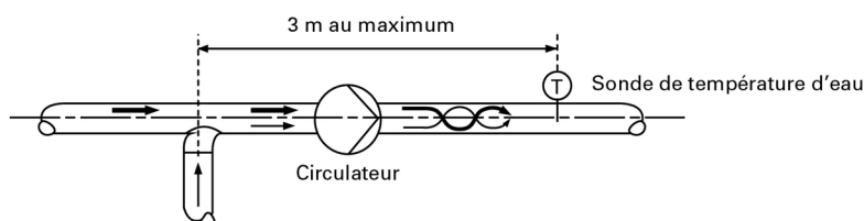
▲ Figure 54 : Montage de la sonde de température d'eau en cas de mélange en amont
