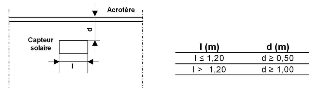
▲ Figure 27 : Implantation de l'équipement – vue en plan
