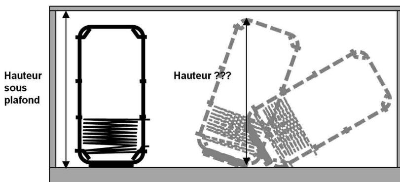
▲ Figure 50 : Contrôle de la diagonale du réservoir
