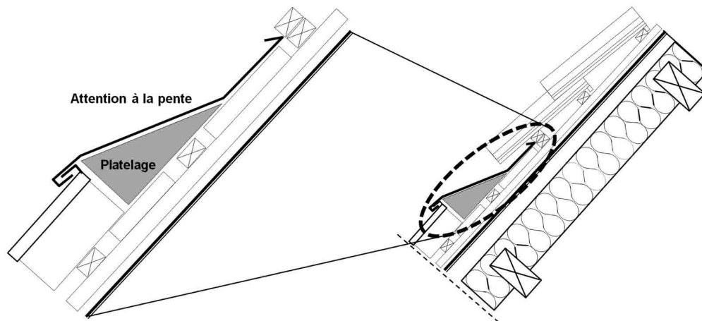
▲ Figure 19 : Exemple de raccordement en tête du capteur avec écoulement des eaux sur le capteur. La pente doit toujours être positive.
