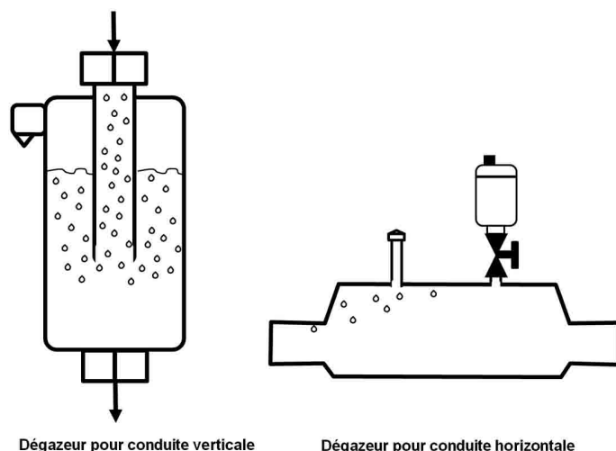
▲ Figure 38 : Exemples de modèles de dégazeur pour canalisations horizontales et verticales
