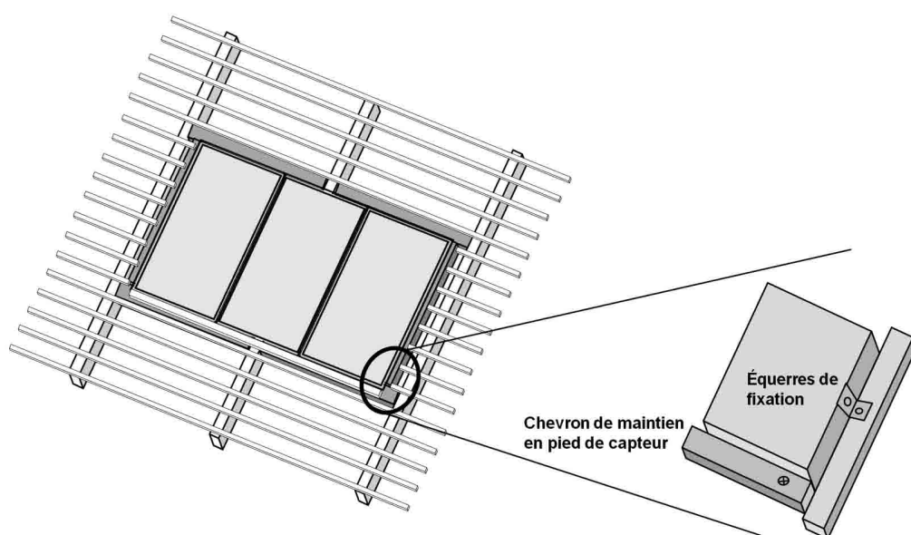
▲ Figure 13 : Capteur incorporé posé sur chevêtre
