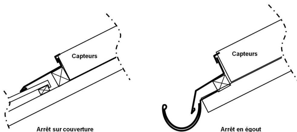
▲ Figure 16 : Exemples de raccordement en pied de capteurs
