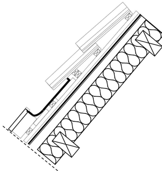
▲ Figure 20 : Exemple de raccordement en tête du capteur avec écoulement des eaux sur les couloirs latéraux
