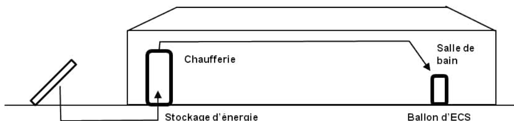
▲ Figure 49 : Implantation du ballon de stockage solaire
