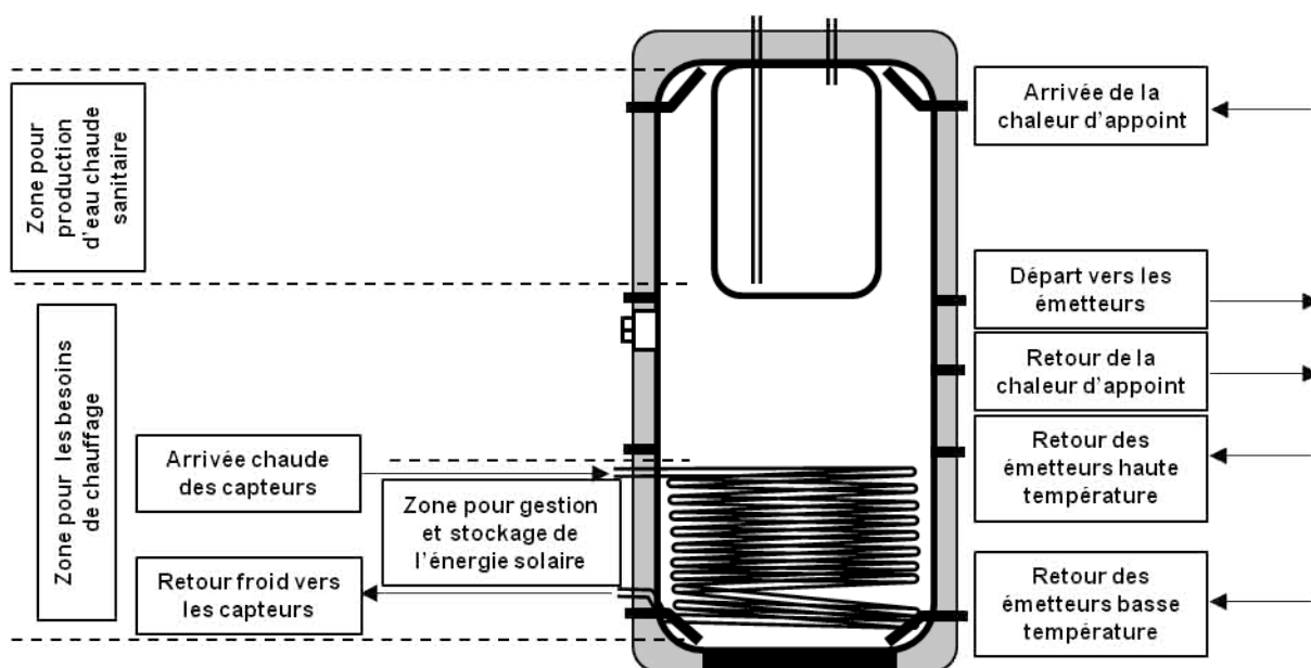
▲ Figure 47 : Représentation des différentes zones d'utilisation d'un ballon de stockage stratifié
