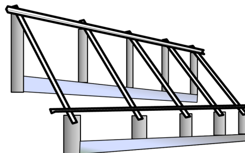
Structure pour capteurs plans avec supports en béton sur talus
