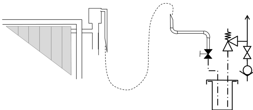
▲ Figure 37 : Purgeur manuel ramené en local technique et branché dans le bidon de récupération
