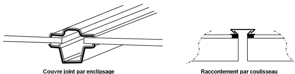
▲ Figure 15 : Différents types de raccordements entre capteurs
