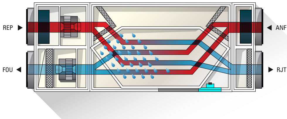
FIGURE 7 Rafraîchissement adiabatique simultané
