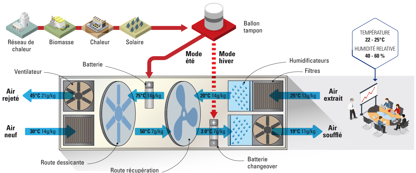
FIGURE 13 Refroidissement adiabatique par roue dessiccante avec systèmes de chauffe
