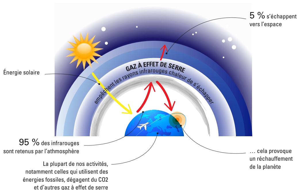
FIGURE 1 Explication du phénomène d'effet de serre
