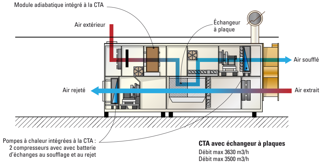
FIGURE 15 Schéma du système mis en place dans la crèche
